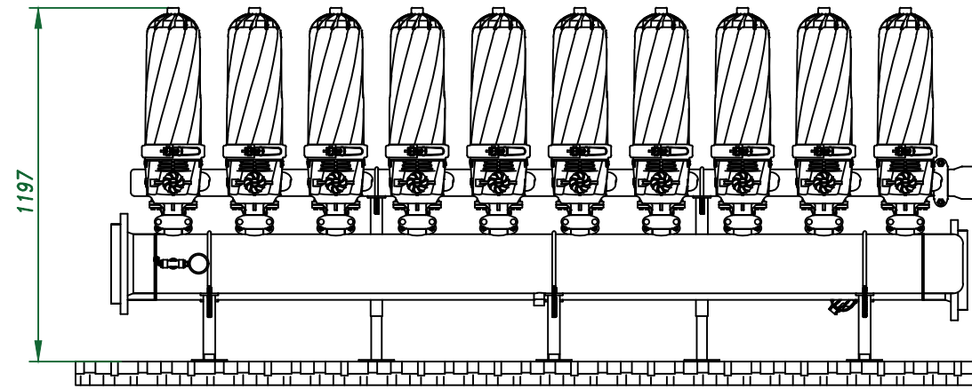
Вид спереди
